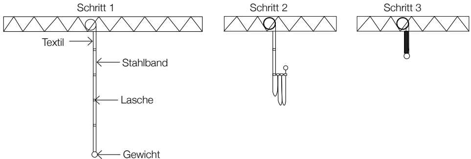
Abbildung: Funktionsweise der Oberrangabtrennung
